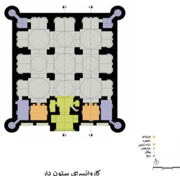
تصویر ۷- پلان کاروانسرای ستون‌دار (Unesco, 2021)
