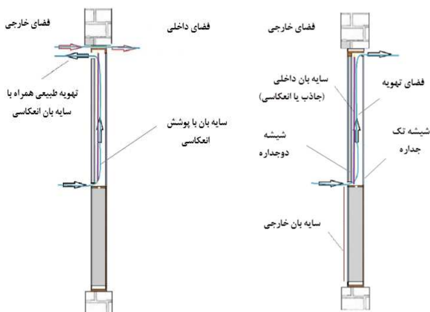
تصویر ۸- ترکیب پنجره‌های هوا گذر با مواد تغییر فاز دهنده (الف) و سایه‌بان داخلی جاذب یا انعکاسی (ب)
