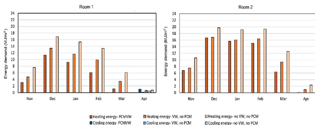
تصویر ۷- تقاضای انرژی ساختمان با سه حالت پنجره به منظور بررسی قابلیت ذخیره سازی انرژی در زمستان
