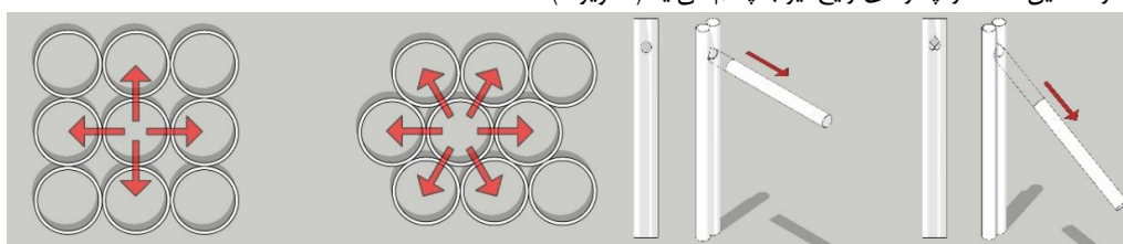
تصویر ۴- تصویر راست: دو نوع از اتصالات لوله‌های مقوایی به یک‌دیگر به وسیله‌ی اتصالات پیچ و مهره؛ تصویر چپ: نحوه‌ی اتصالات در حالت راست گوشه و زاویه‌دار
