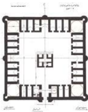
تصویر ۲- کاروانسرای بدون رواق، کاروانسرای قلعه سنگی رباط کریم (هیلن براند، ۱۳۸۹)
