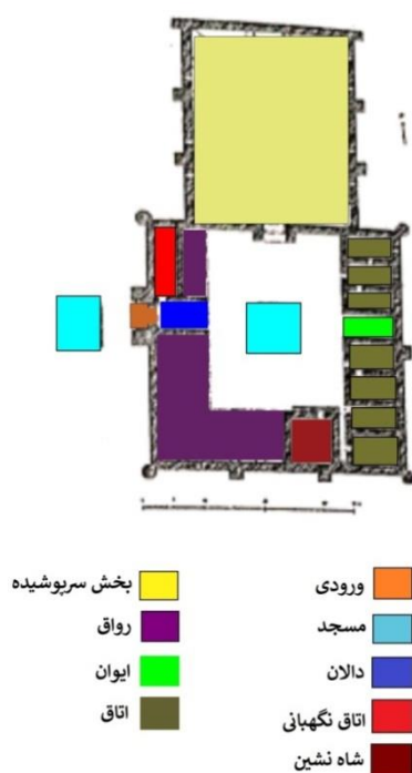
تصویر ۱۱- جانمایی فضاها در یک نمونه از کاروانسراهای سلجوقی آناتولی
