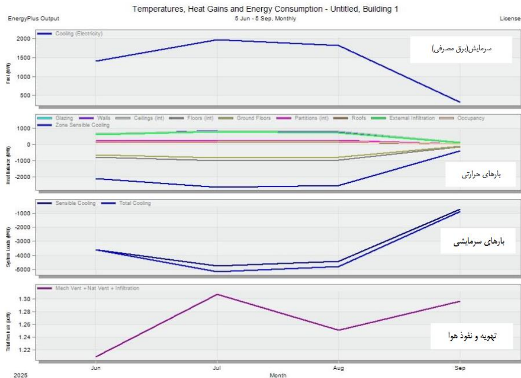
تصویر ۵- سرمایش (kWh)، بارهای حرارتی ۶ (W) و سرمایشی ۷ (W)، تهویه و نفوذ هوا ۸ (ACH) در ساختمان عایق شده
